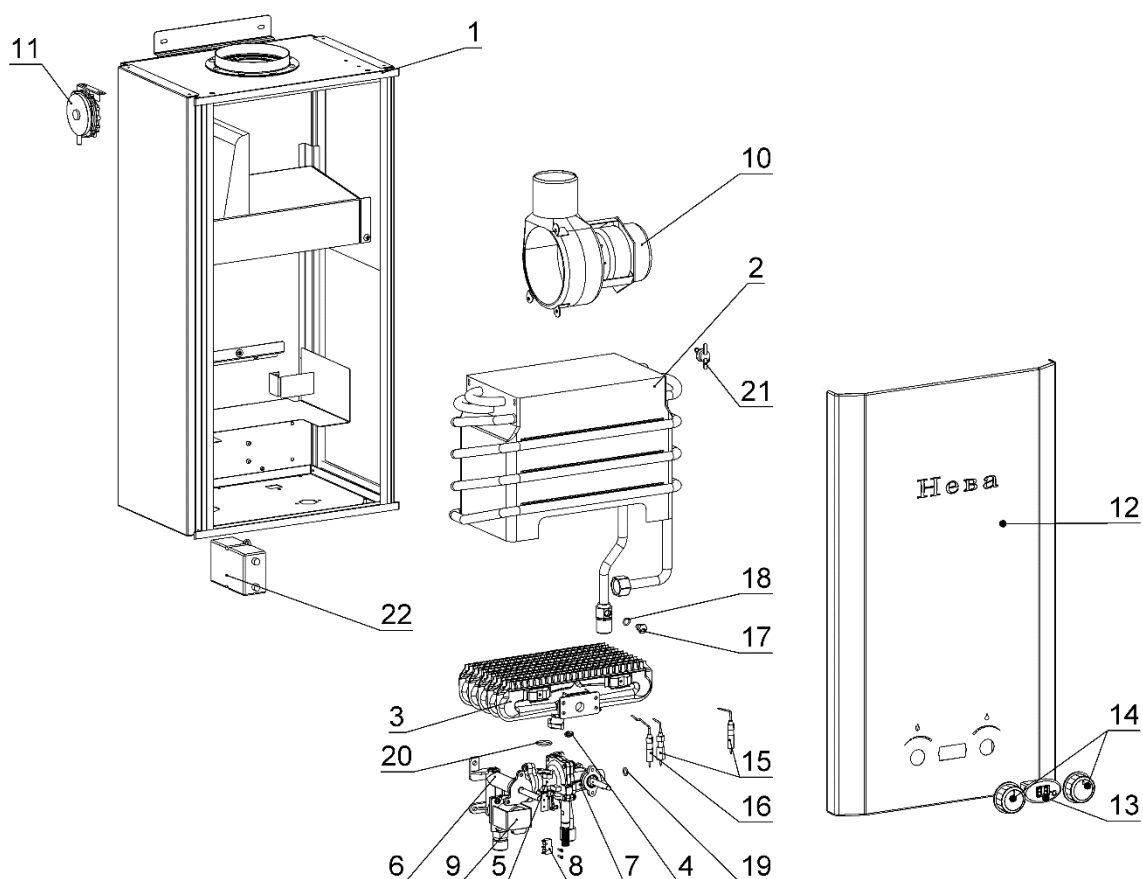
Рисунок 9. Вид аппарата с разнесёнными частями
